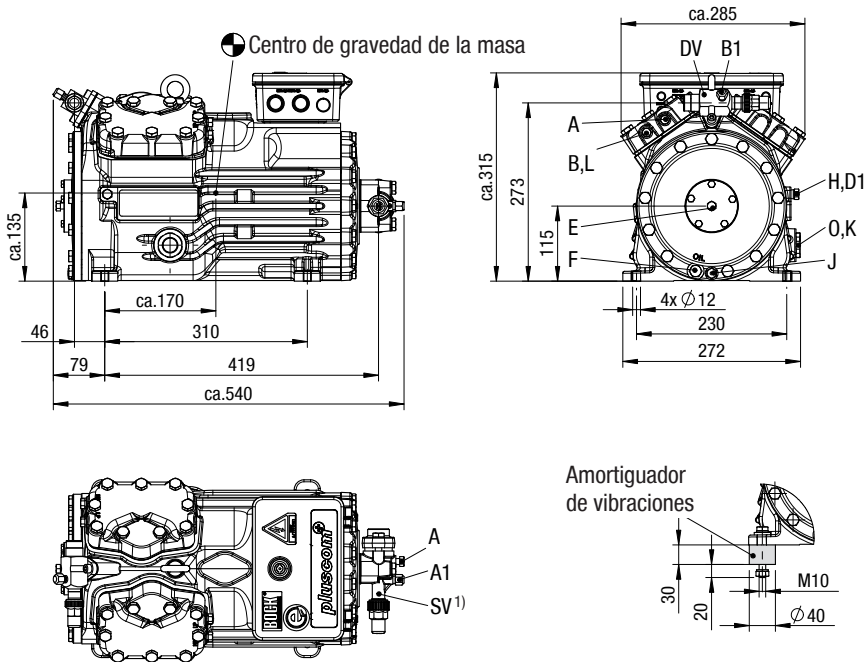
Medidas en mm Fig. 22
