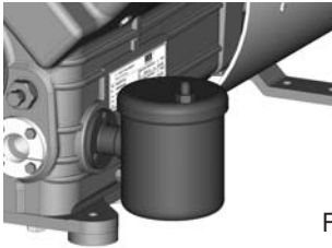
Regulador mecánico del nivel de aceite en la conexión "0"
